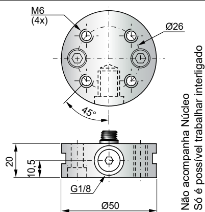
PNB-100-050 - Base de Interligação
